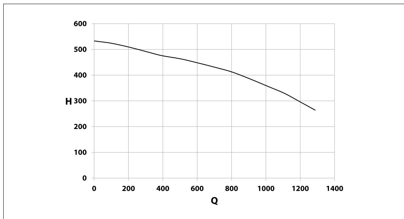
Рис. 15 Располагаемый напор
