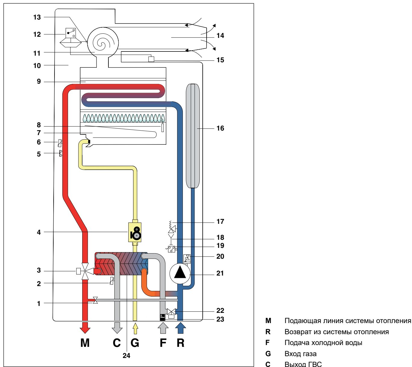
Рис. 4 Гидравлические схемы
