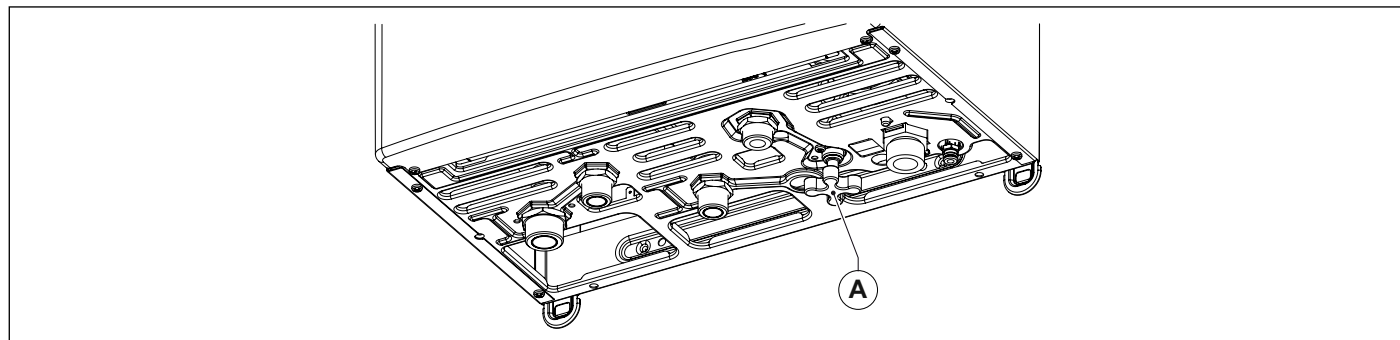
Рис. 2 Кран заполнения
