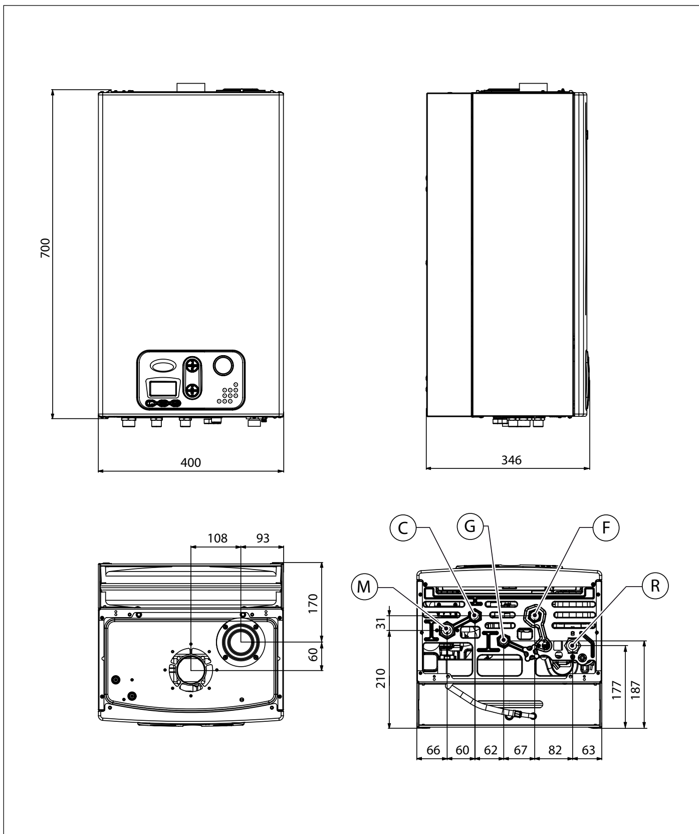
Рис. 3 Габаритные размеры
