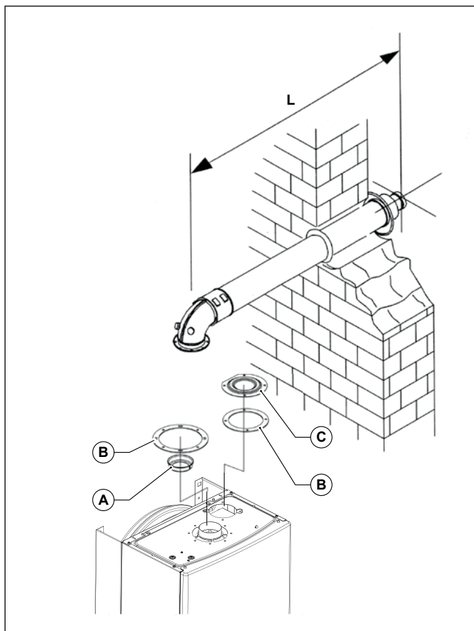
Рис. 6 OKITCONC00 (100/60 мм)
